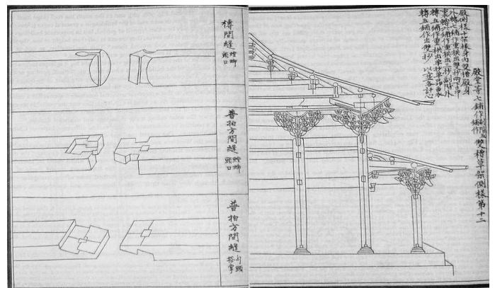
Trabajos de espiga y mortaja de vigas de unión y vigas transversales, Yingzao Fashi
